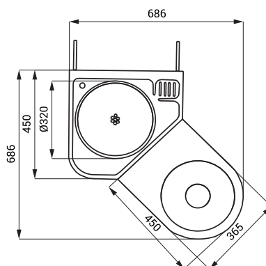
SLWN 08PP/ZPP
