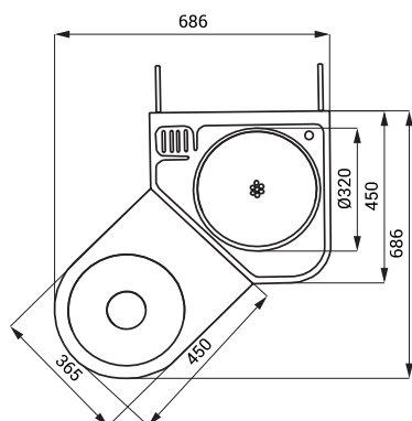
SLWN 08LP/ZLP
